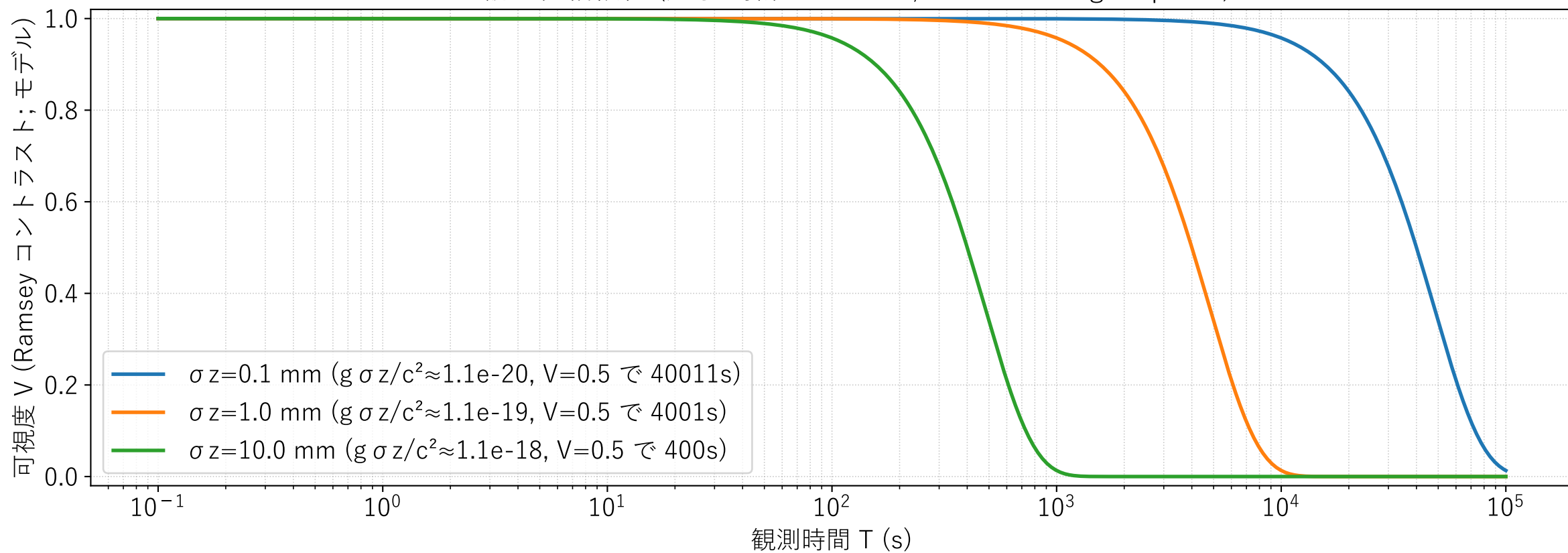
重力誘起位相緩和 (光学 時計 ensemble; Gaussian height spread)
