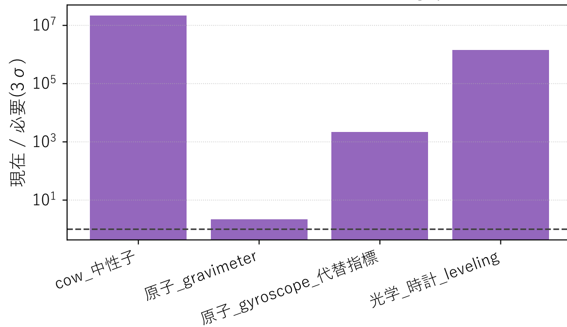
原子-interferometer 精密 gap
