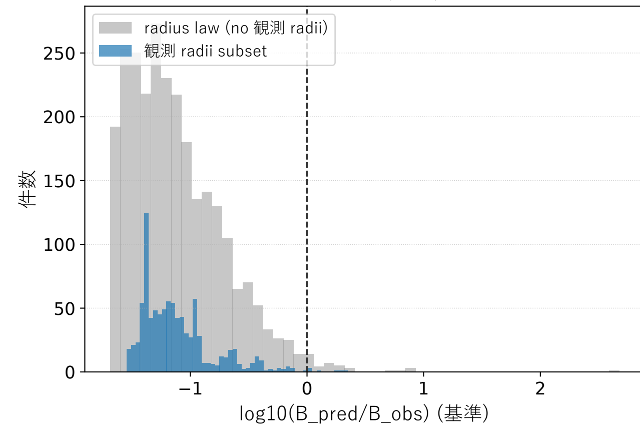
残差 分布 (基準)
