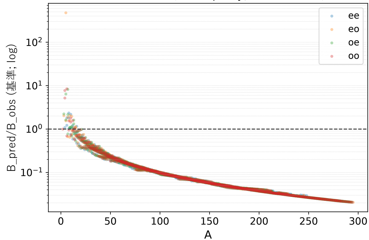
基準 残差 vs A (color=parity; ee/eo/oe/oo)
