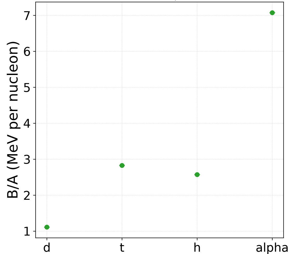
束縛エネルギー per nucleon
