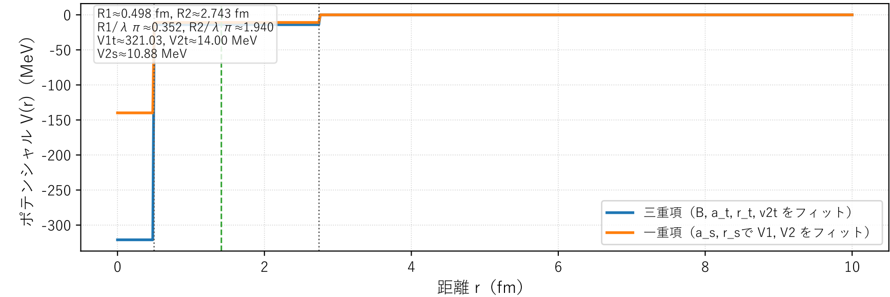
eq19 (Nijmegen) \lambda \pi 拘束2レンジ: 三重項をフィットし、一重項(a_s,r_s)を符号付きV2でフィット 2レンジ ( \lambda \pi 拘束、符号付きV2_s)
