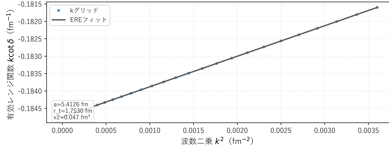
三重項: EREフィット (v2を目標)
