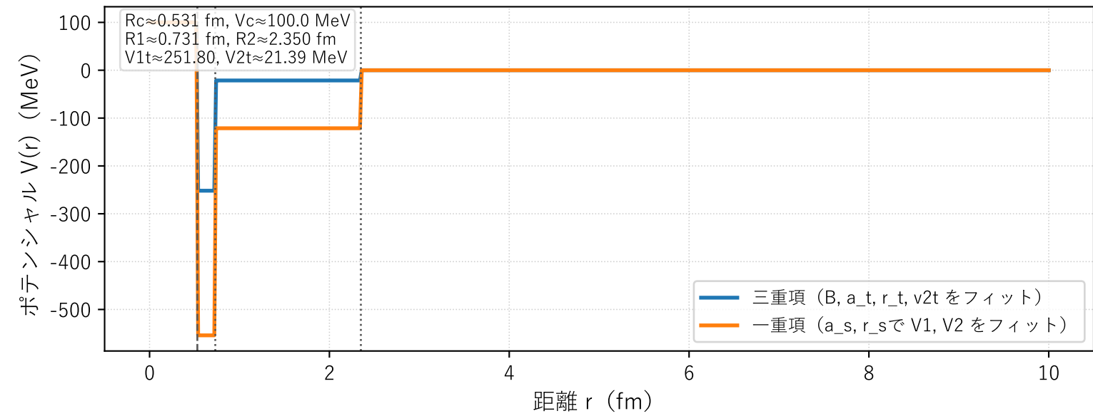
eq18 (GWU/SAID) 反発コア + 2レンジ井戸
