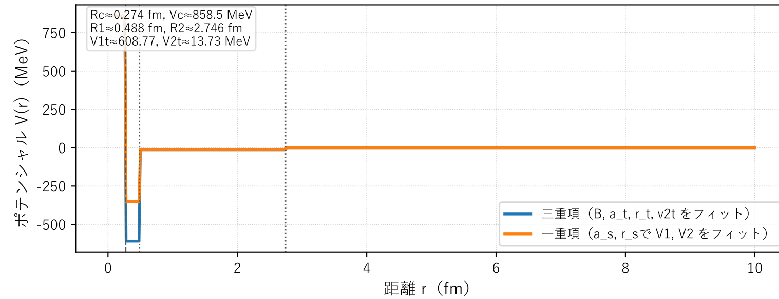
eq19 (Nijmegen) 反発コア + 2レンジ井戸
