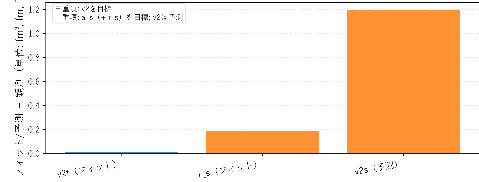
観測値とのクロスチェック (eq出典)
