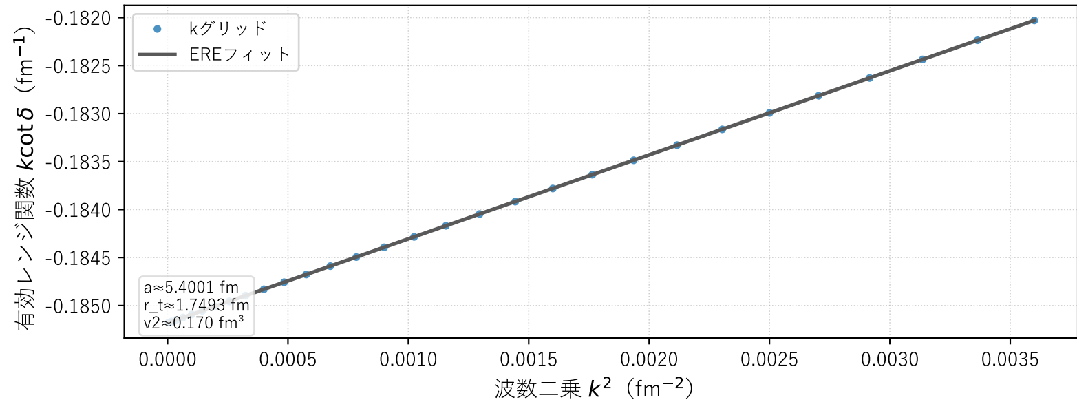
三重項: EREフィット (v2を目標)
