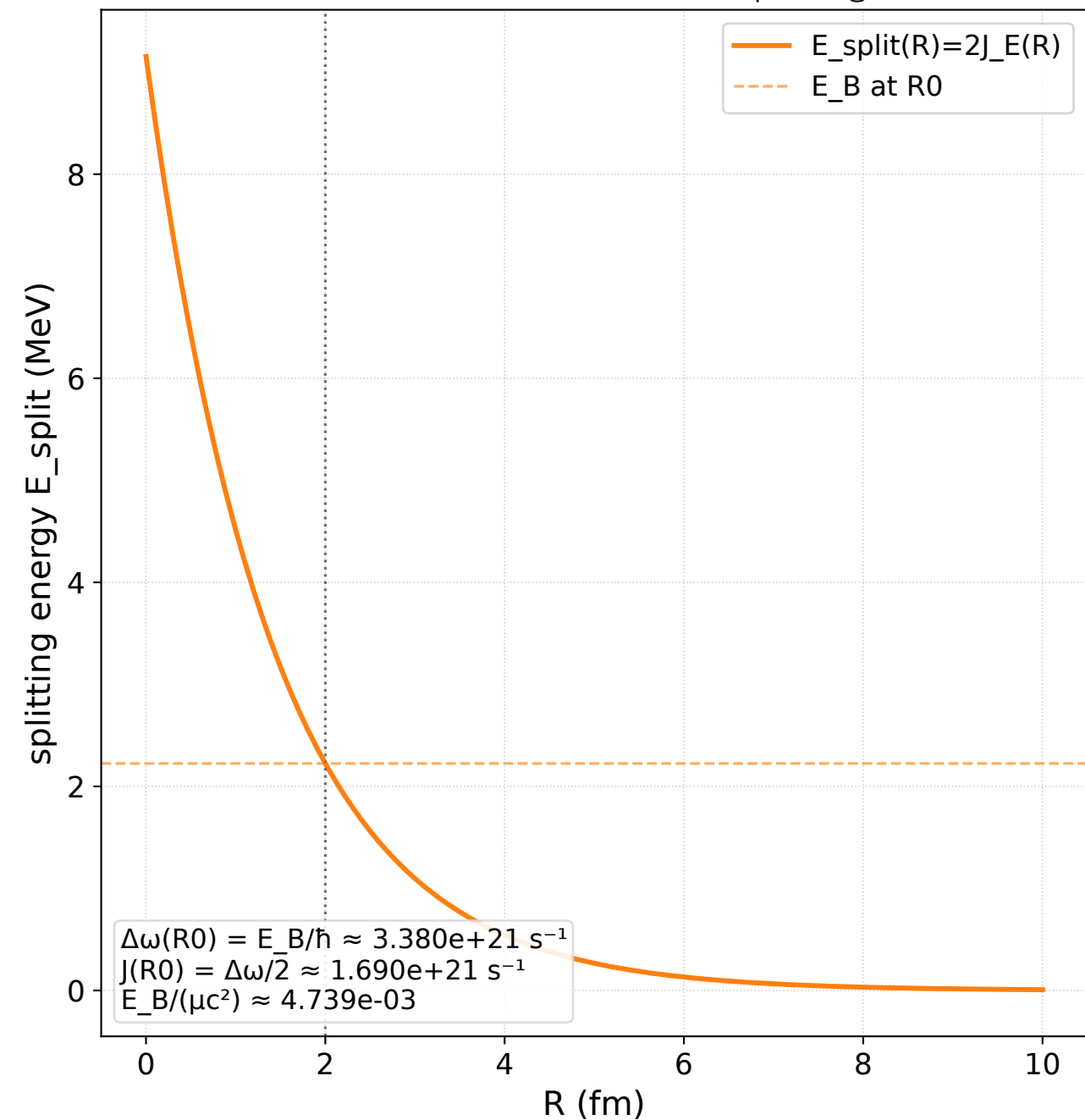
束縛スケール from mode splitting
