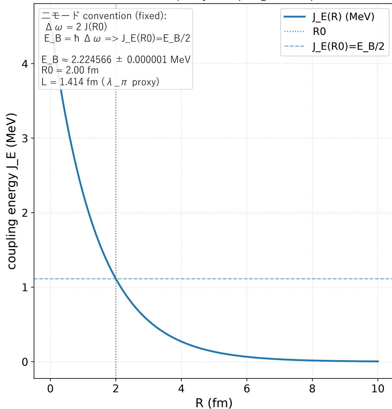
近接場 干渉 proxy: coupling envelope
