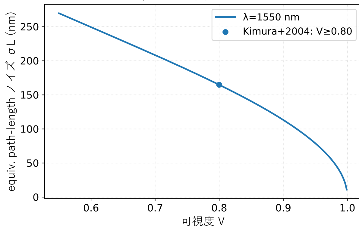
単一光子 干渉: V \rightarrow \sigma L
