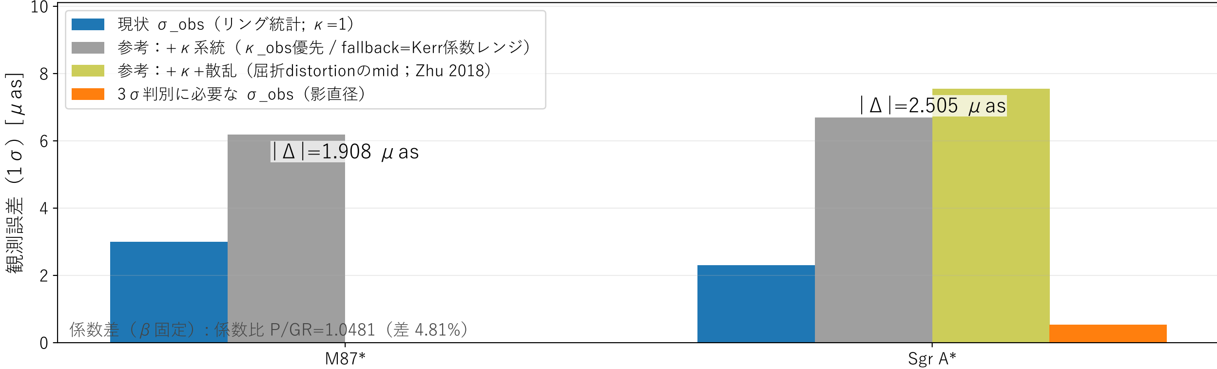
EHT（ブラックホール影）：差分予測を3 \sigma で判別するための必要精度（ \kappa /散乱は参考）
