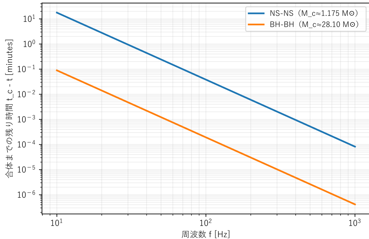
重力波：chirp のスケーリング（四重極）
