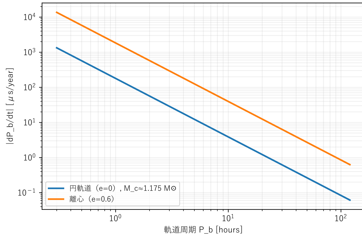
二重パルサー：軌道減衰のスケーリング（四重極）
