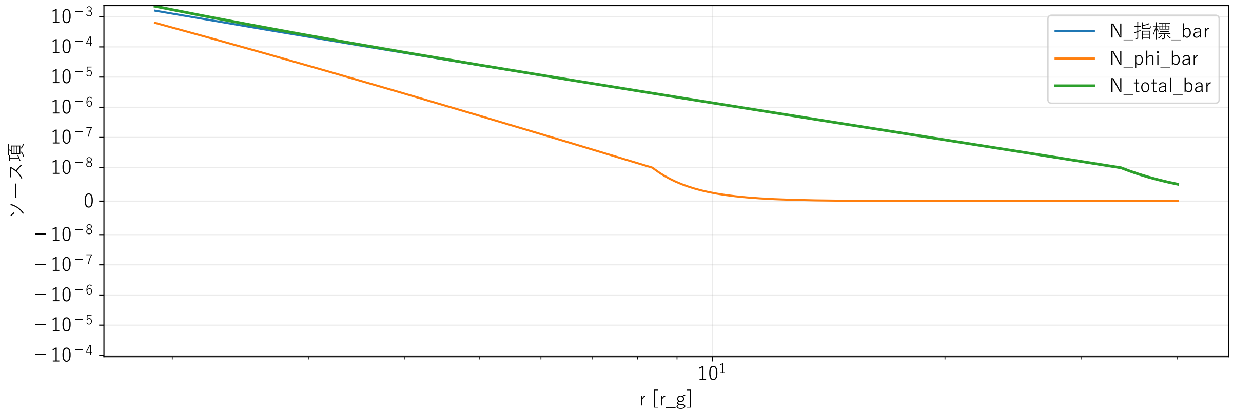
N0^(2) の球面平均
