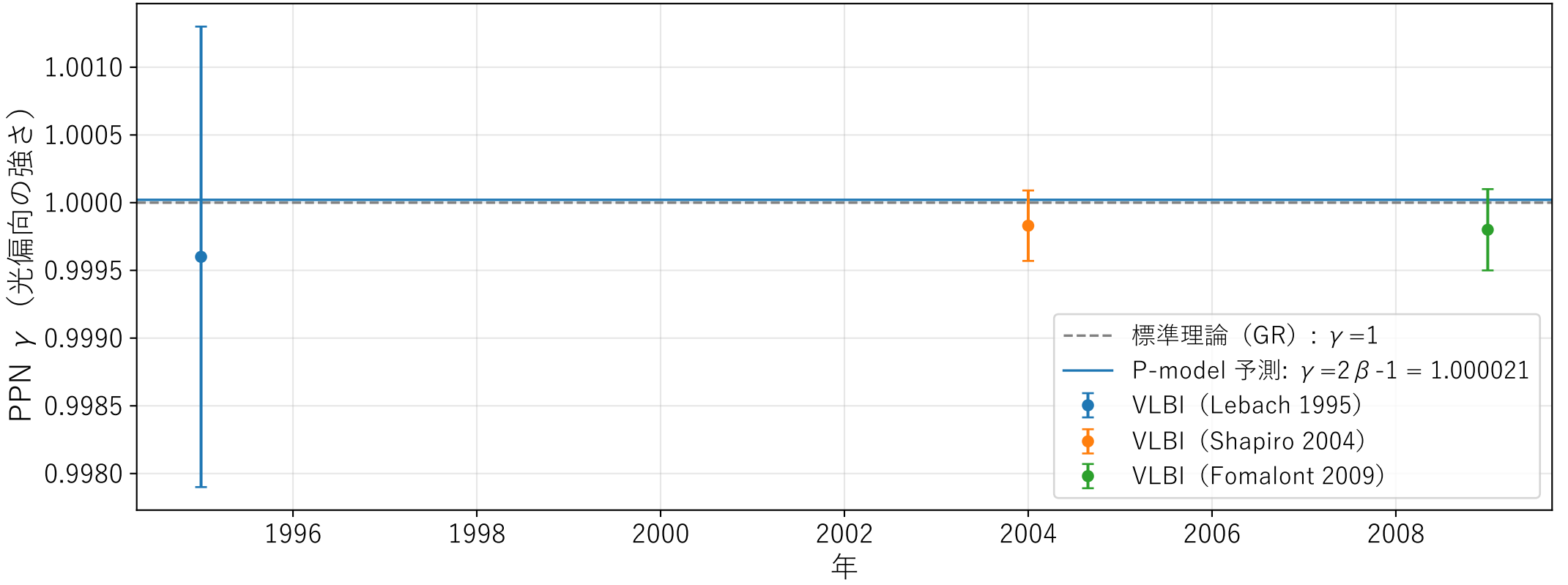
光偏向パラメータ \gamma （観測）
