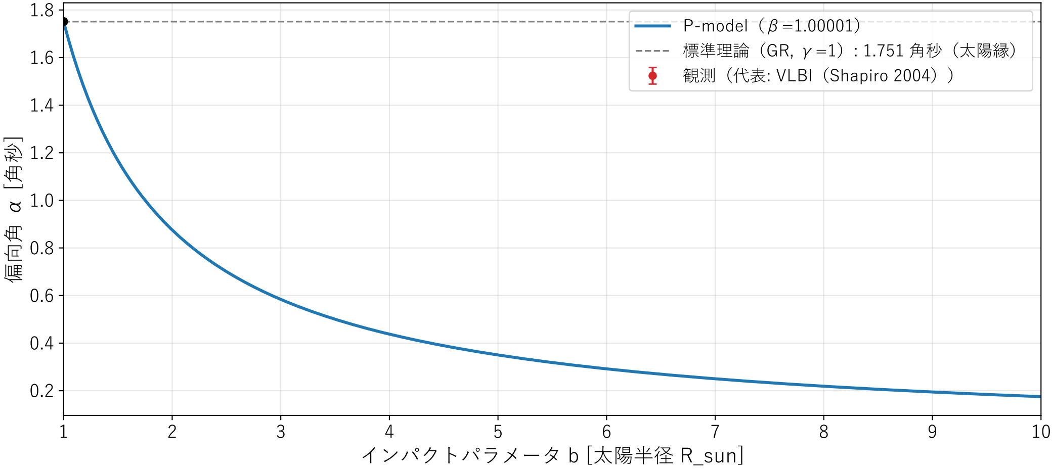
太陽重力による光の偏向（弱場）
