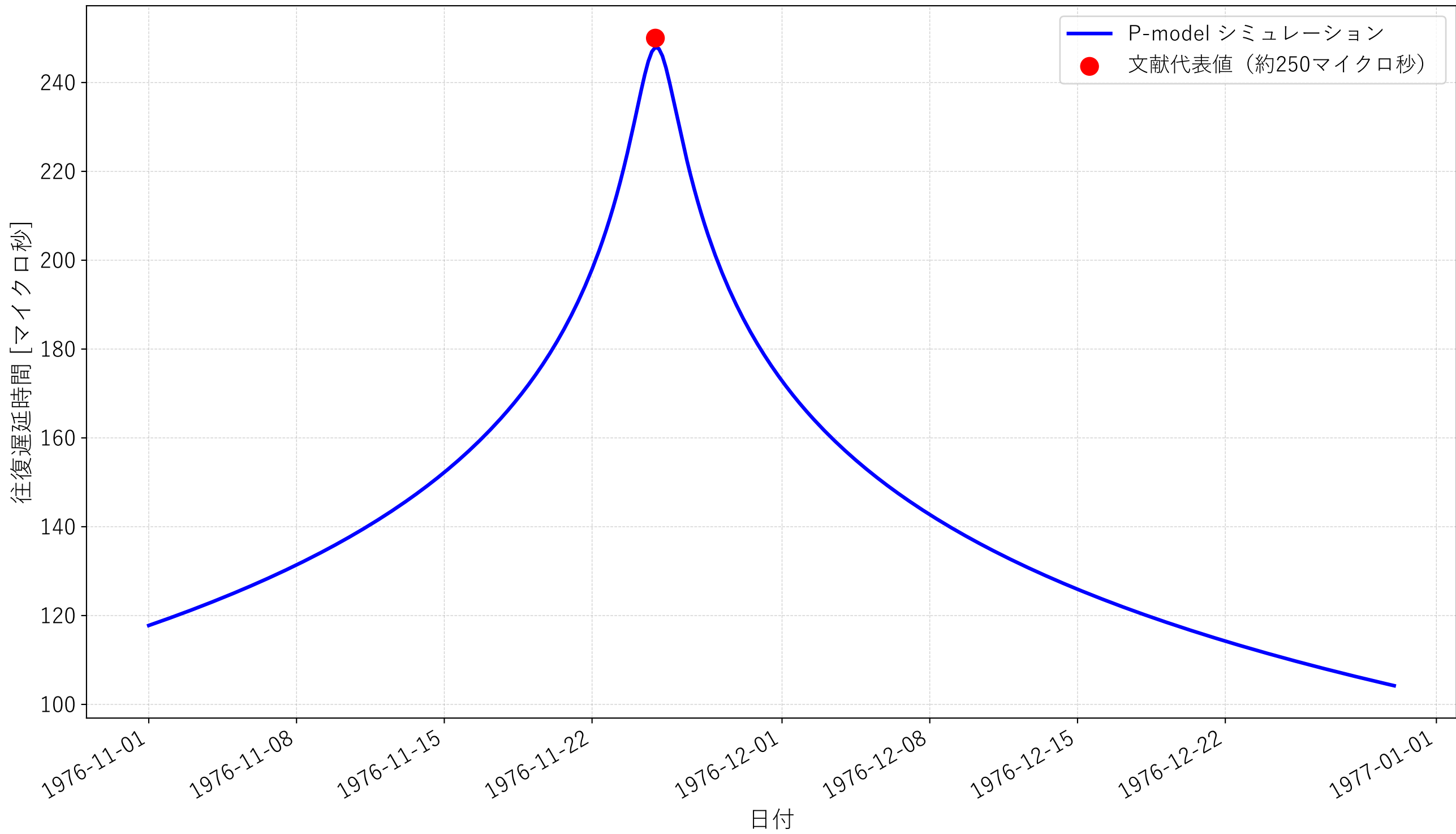
バイキング 太陽合（1976）：P-model シミュレーション vs 文献代表値
