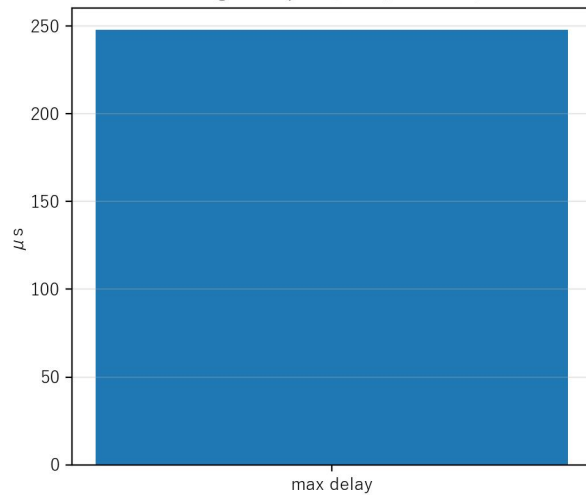
Viking : Shapiro遅延 (理論最大)
