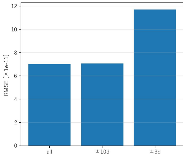
Mercury : 近日点移動 (比較)
