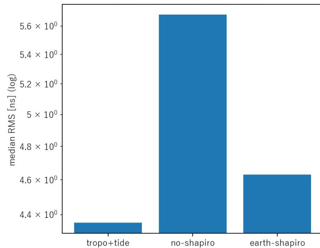
LLR : 中央値RMS (モデル差)
