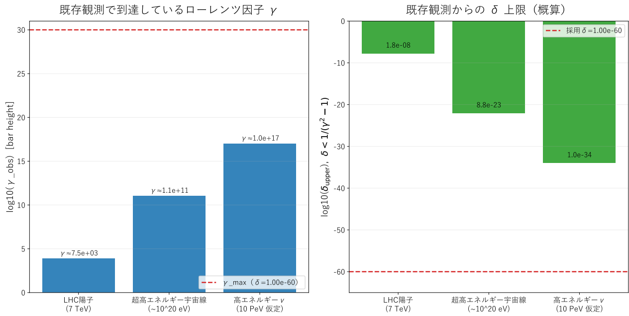
図 5: 速度飽和パラメータ \delta の制約図。既存観測が到達するローレンツ因子 \gamma に基づく上限を並置し、許容レンジのオーダーを比較する。
