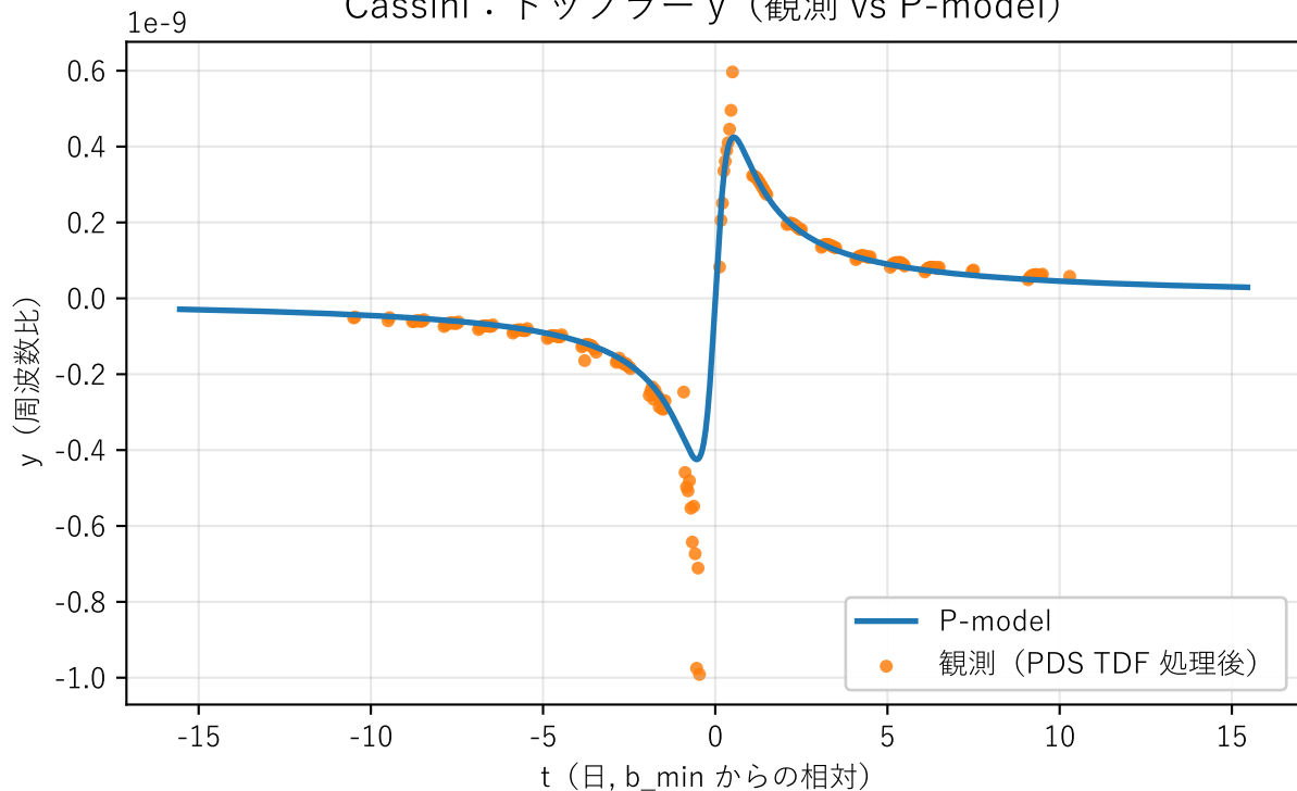
Cassini : ドップラー y (観測 vs P-model)
