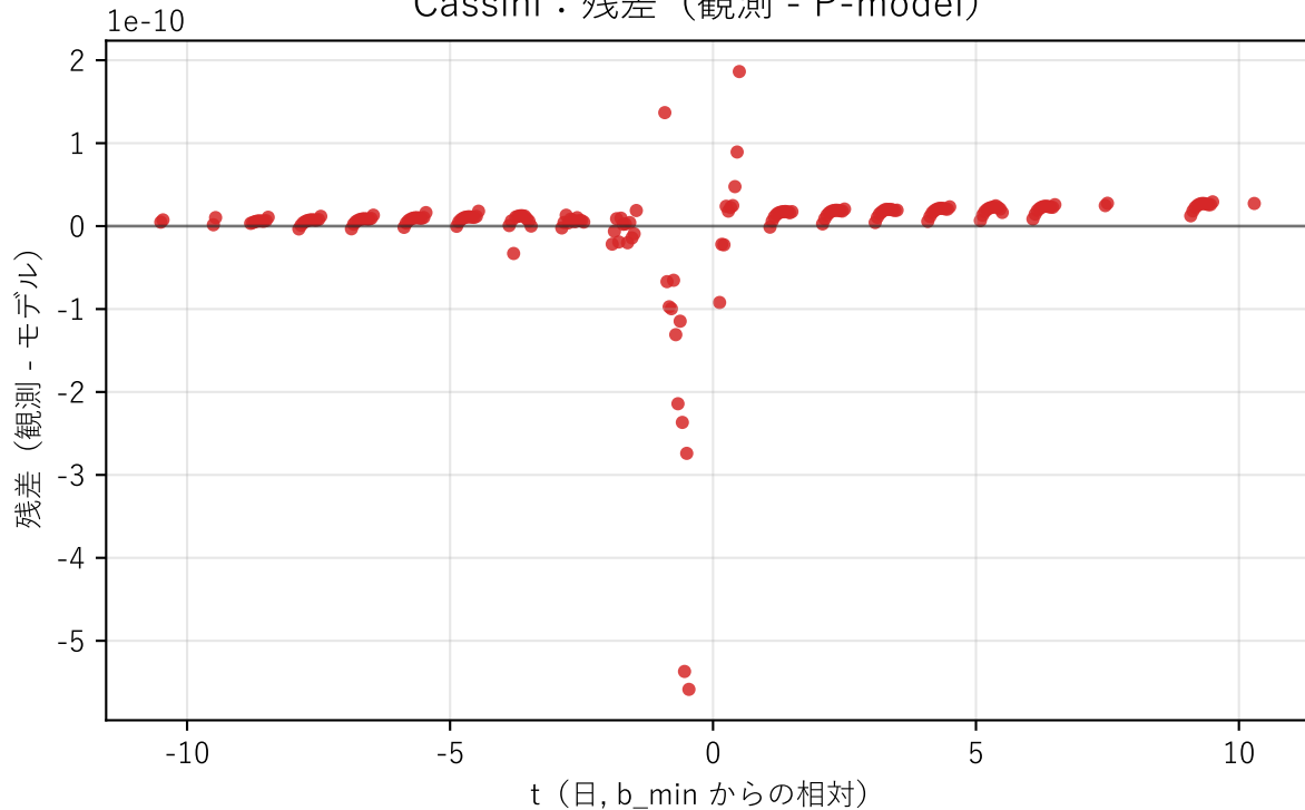
Cassini : 残差 (観測 - P-model)
