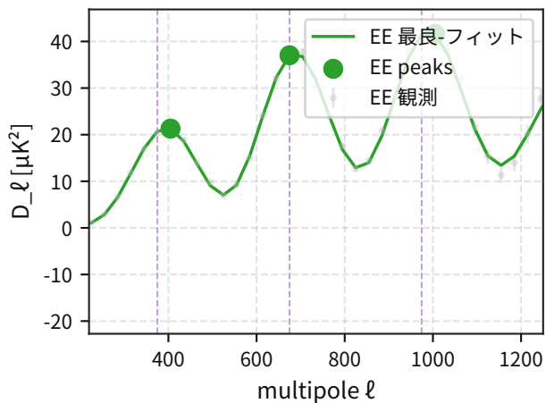
位相ずれ監査 (Planck TT/TE/EE)
