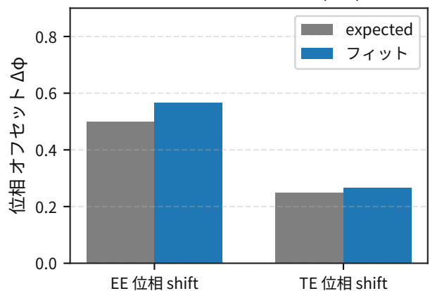
位相ずれ監査 (Planck TT/TE/EE)
