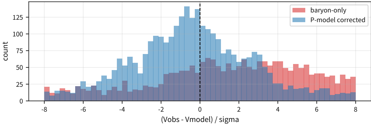
正規化残差分布
