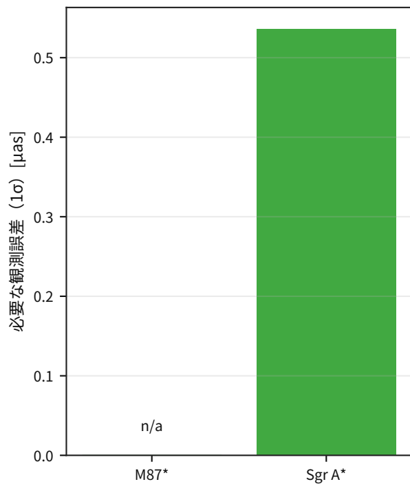
3\sigma で判別するための必要精度
