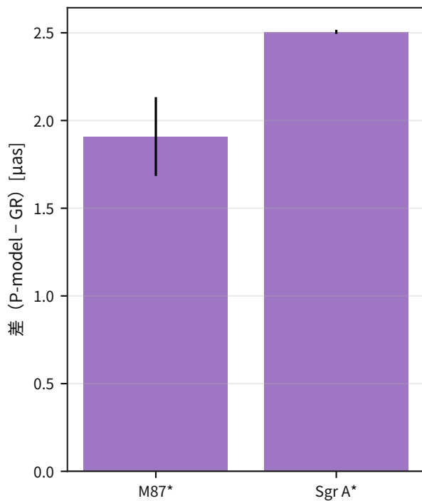
差分予測：シャドウ直径の差
