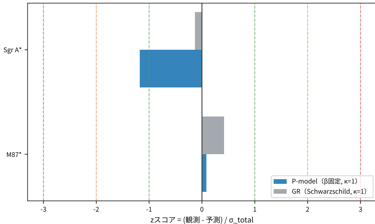
EHT：観測とモデルのずれ (zスコア, \kappa=1 )
