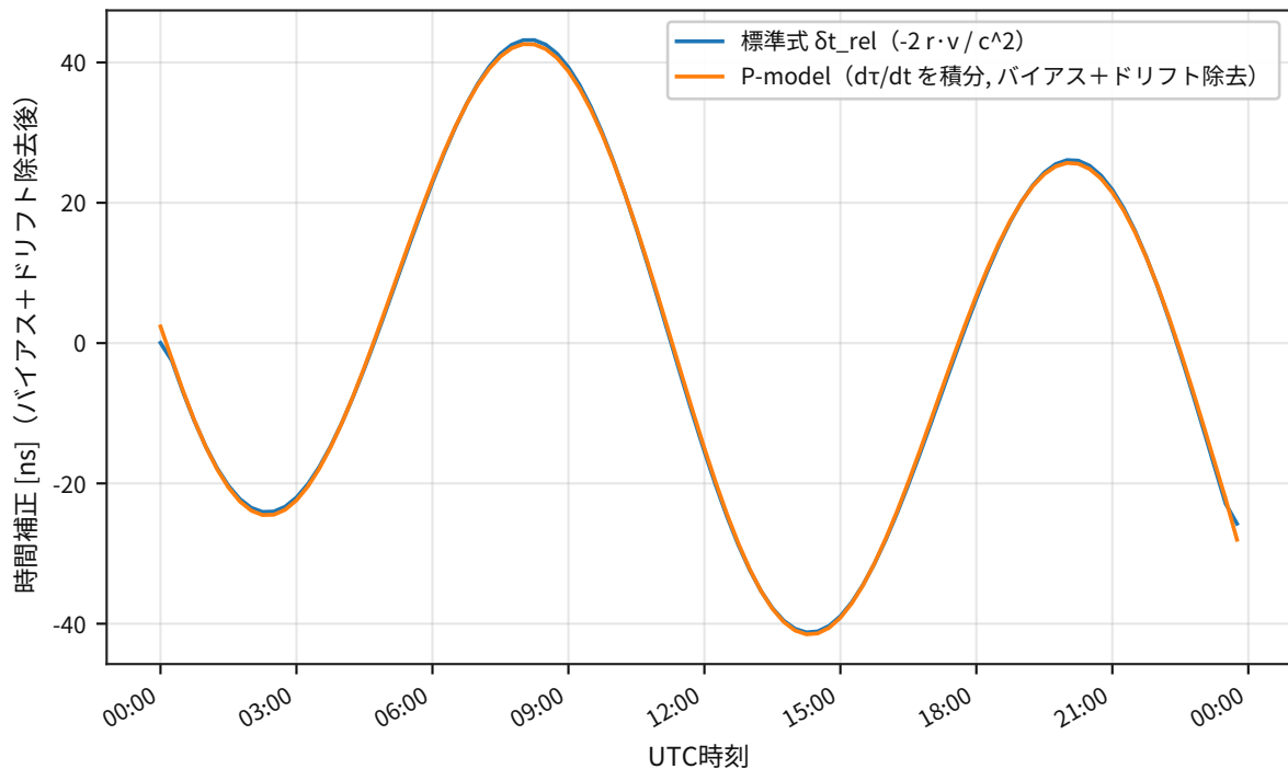
GPS: 相对補正 (近日点効果) G02
