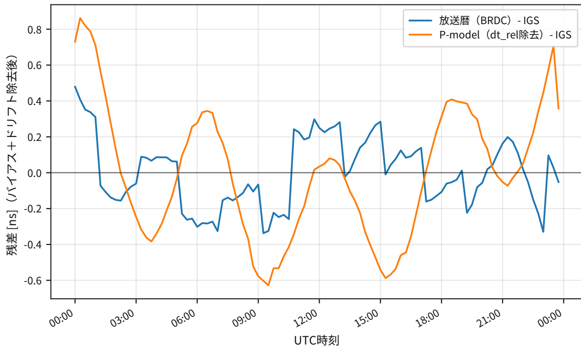
GPS 時計残差: G01 (観測 IGS に対する比較)
