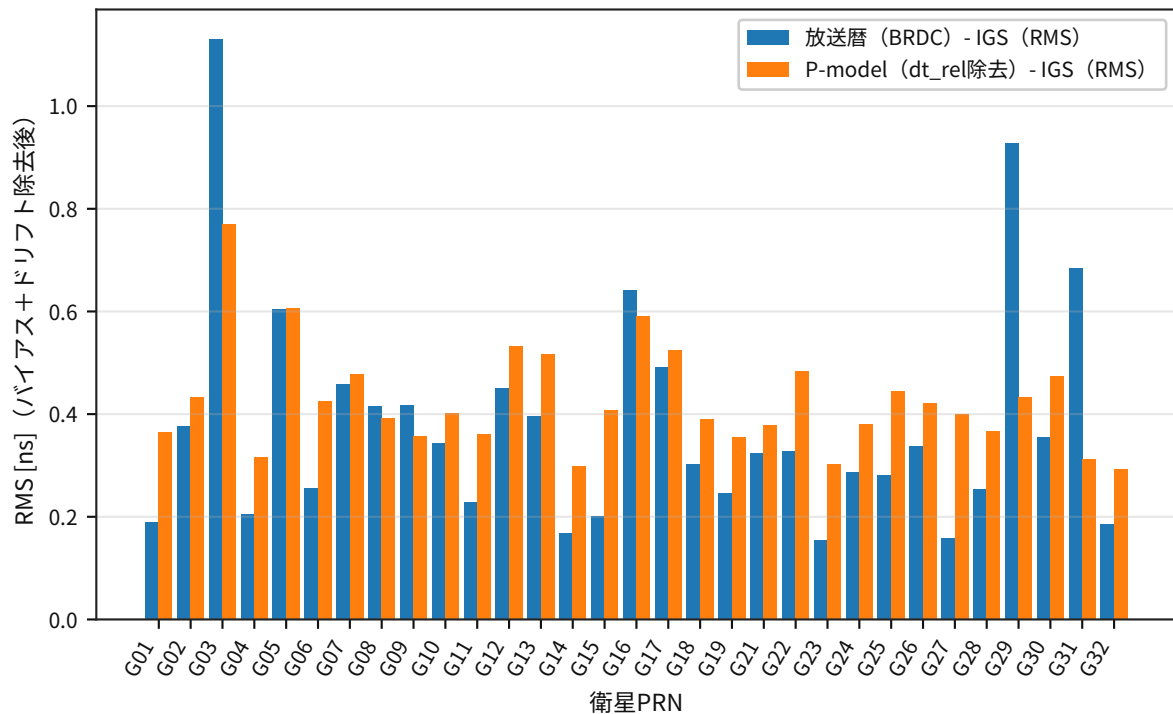
GPS: 観測 IGS に対する残差 RMS (全衛星)
