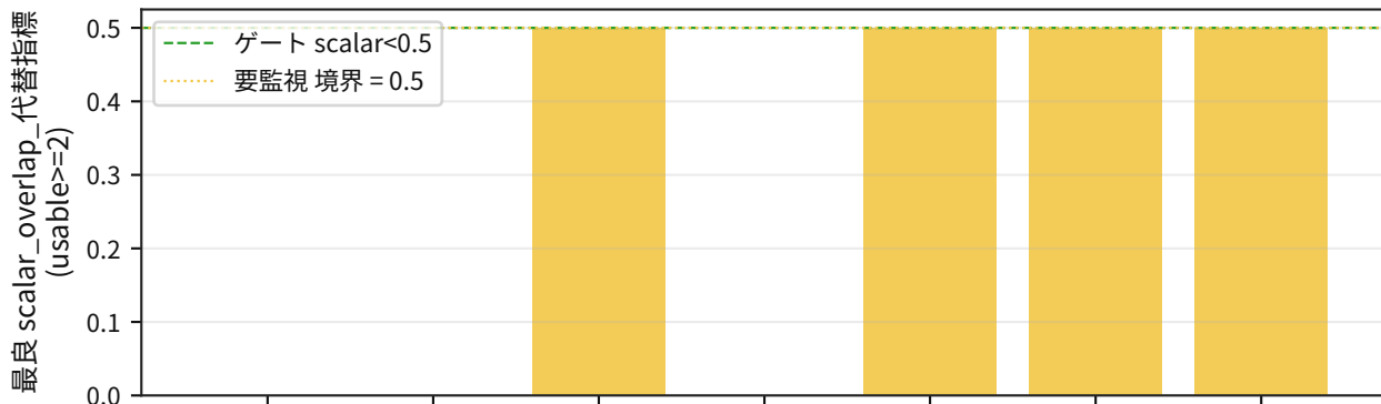
GW偏光カバレッジ拡張監査 (部分集合 掃引)
