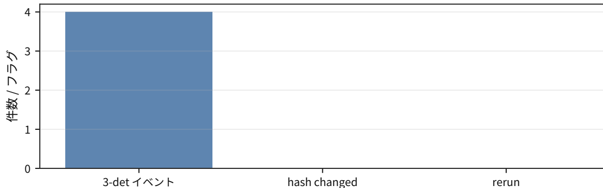
GW偏光イベント更新ウォッチ (3-detector)
