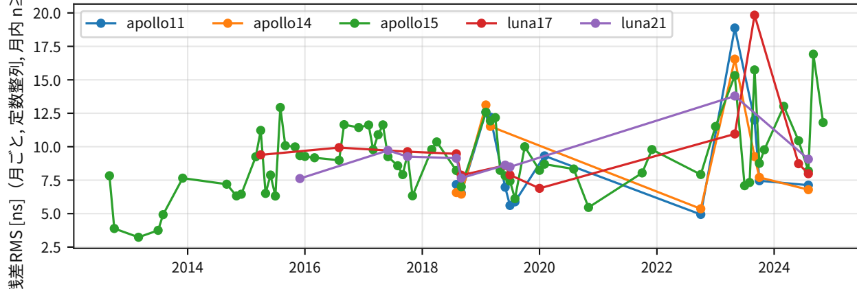
月レーザー測距 (LLR: Lunar Laser Ranging) : GRSM 残差RMS (反射器別の期間依存, 月内 n \geq 30 のみ表示)
