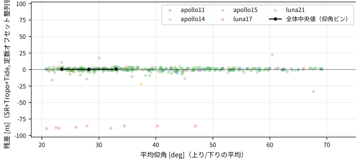
月レーザー測距（LLR: Lunar Laser Ranging）：MATM 残差と仰角（低仰角での系統誤差の有無を確認）
