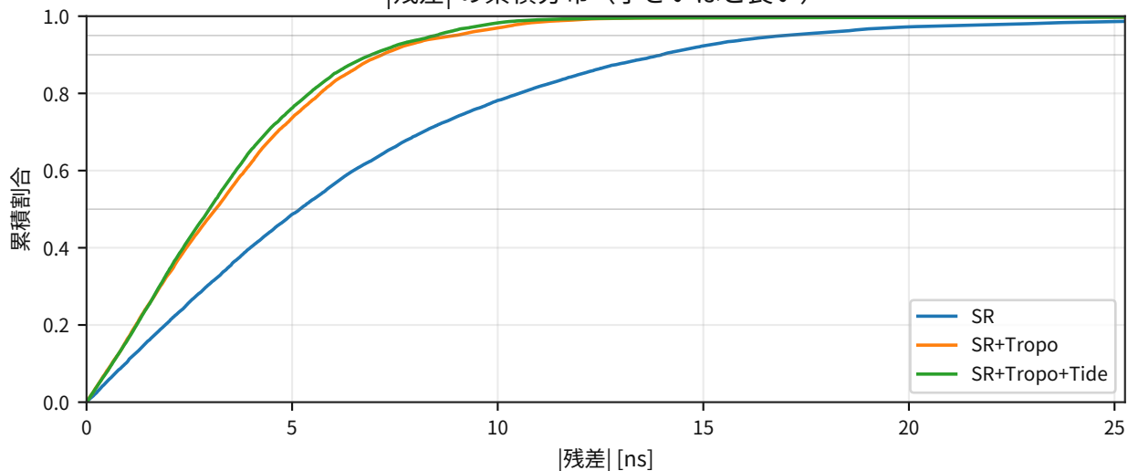
|残差|の累積分布（小さいほど良い）
