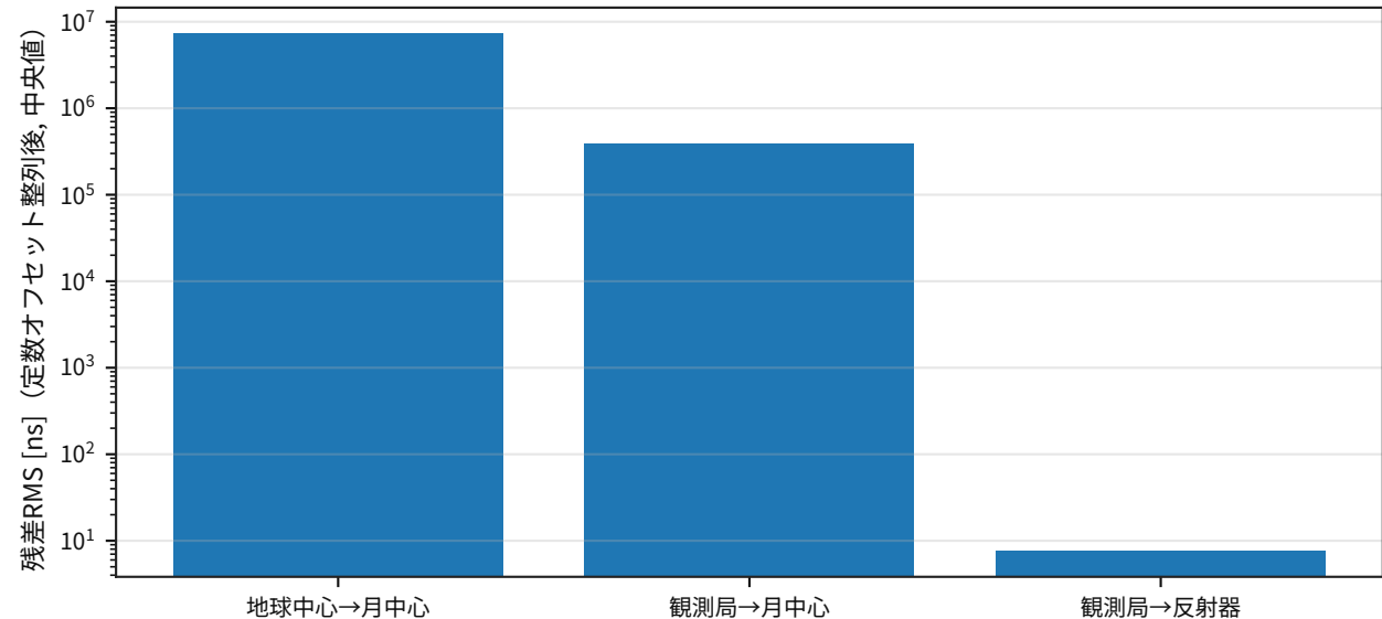
月レーザー測距（LLR: Lunar Laser Ranging）：モデル改善の効果（全グループ中央値）
