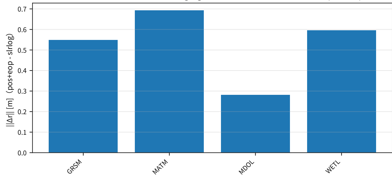
月レーザー測距（LLR: Lunar Laser Ranging）：局座標の差分（一次ソースpos+eopの影響）
