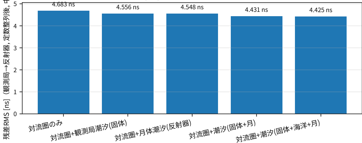
月レーザー測距 (LLR: Lunar Laser Ranging) : 潮汐の寄与 (固体潮汐/海洋荷重/月体潮汐, 対流圏あり)
