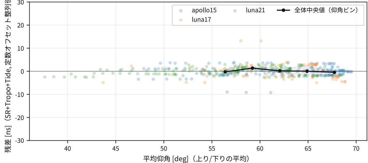
月レーザー測距（LLR: Lunar Laser Ranging）：WETL 残差と仰角（低仰角での系統誤差の有無を確認）
