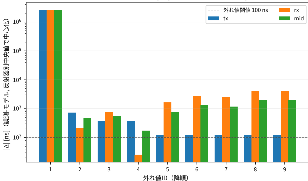
月レーザー測距（LLR: Lunar Laser Ranging）：外れ値の time-tag 感度（tx/rx/mid）
