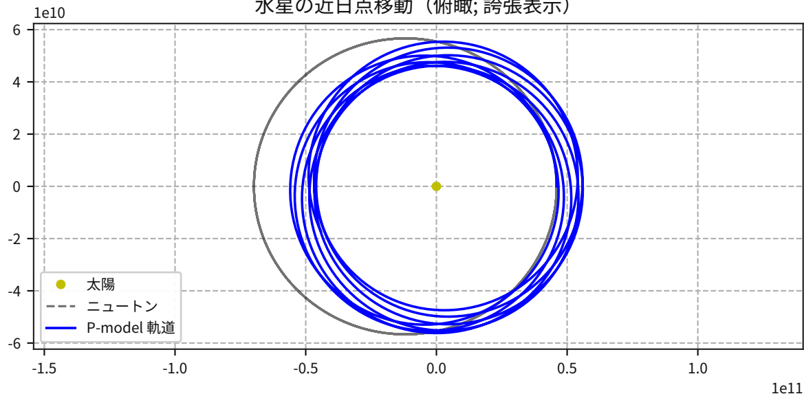
水星の近日点移動（俯瞰; 誇張表示）
