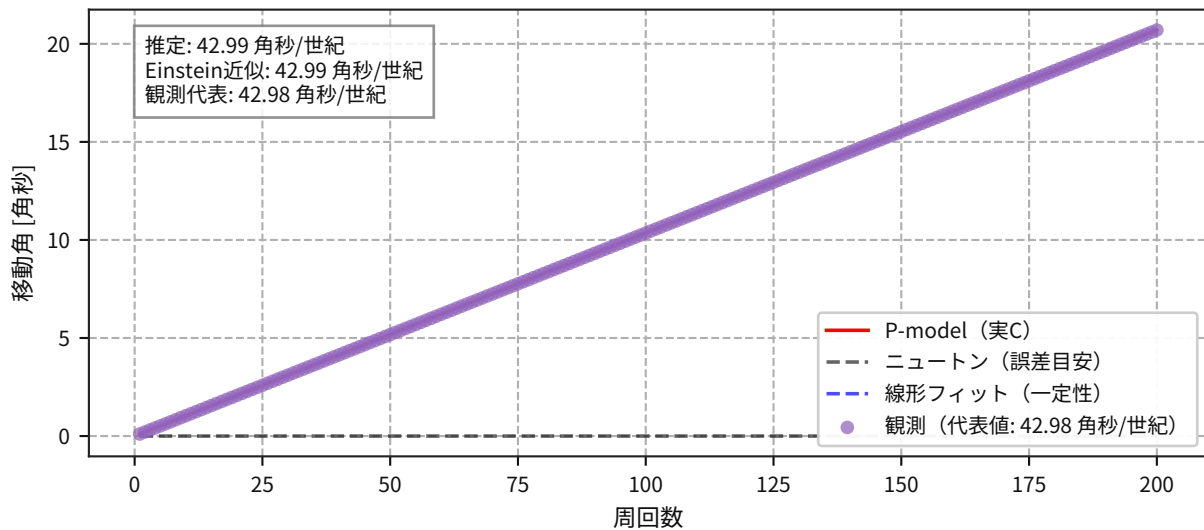
近日点移動の累積（実C）
