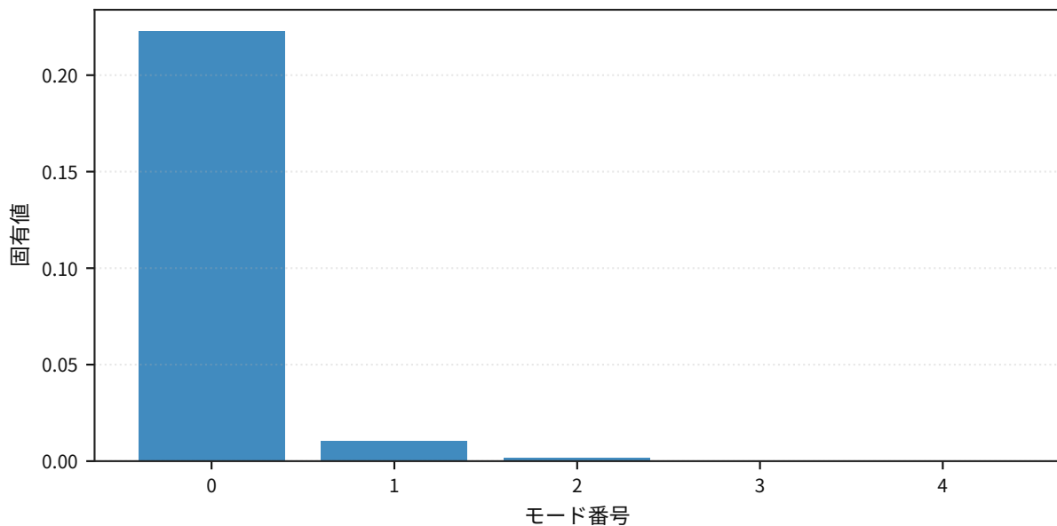
共分散 固有値s
