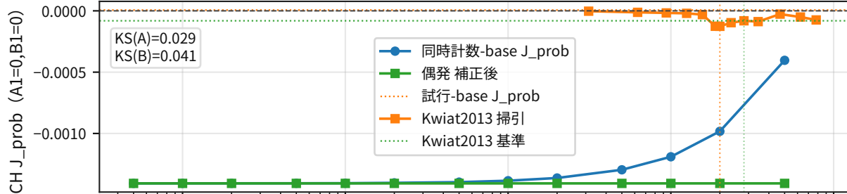
NIST : CH J_prob と窓幅
