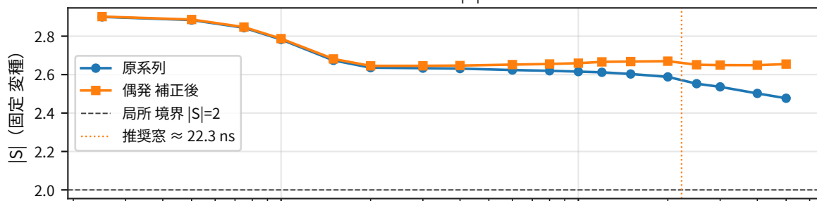
Weihs 1998 : |S| と窓幅
