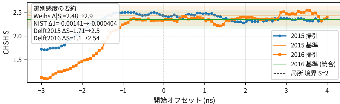
Delft : CHSH S と開始オフセット
