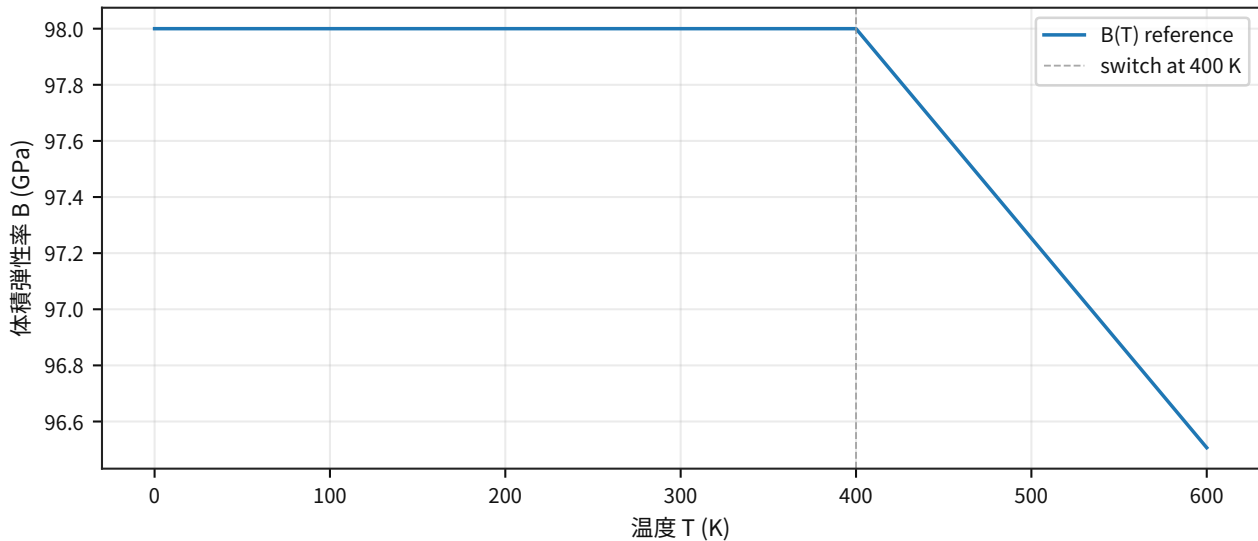
シリコン 体積弾性率 B(T) (Ioffe elastic constants reference)
