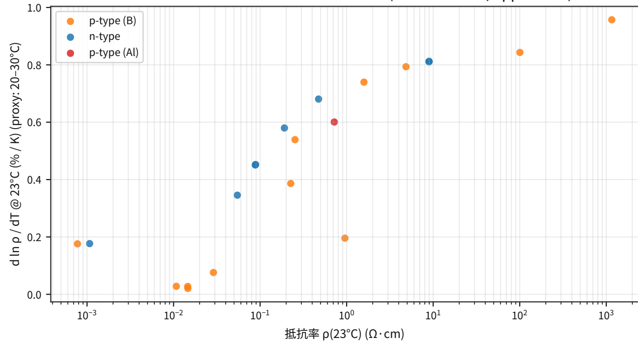
シリコン 抵抗率 温度係数 near room 温度 (NBS IR 74-496; Appendix E)
