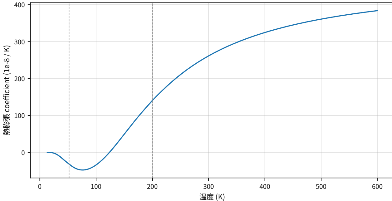
Si 熱膨張 coefficient (NIST TRC fit)
