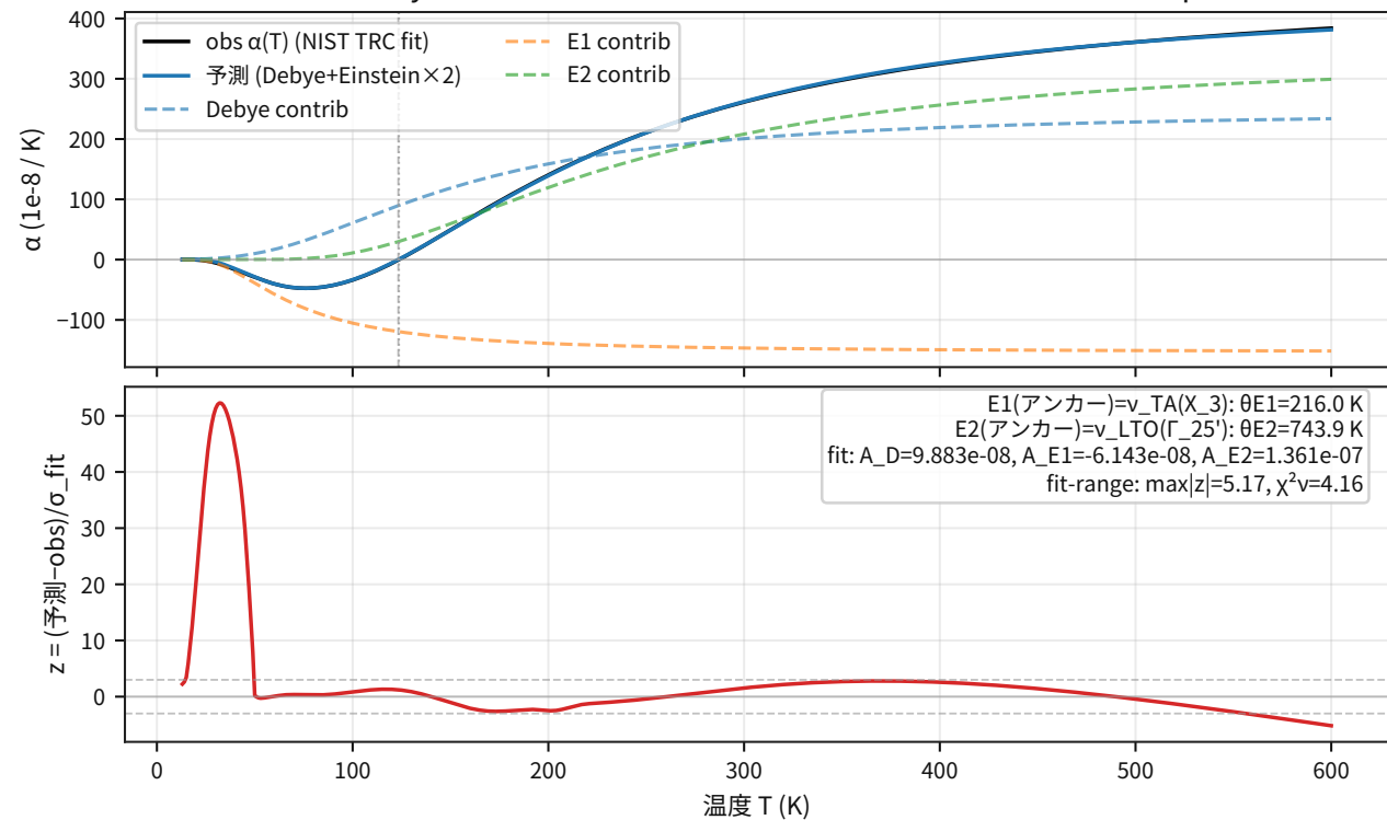
Si 熱膨張: Debye+Einstein×2 with \theta_E anchors from Ioffe フォノン frequencies
