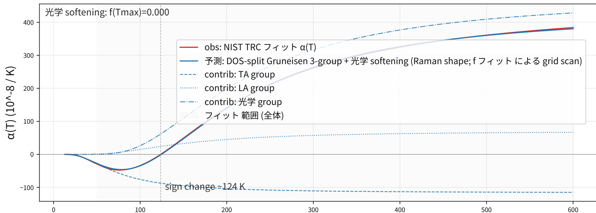
Si 熱 拡張: フォノン DOS constrained Gruneisen チェック
