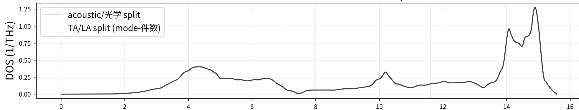
Si フォノン DOS 代替指標 (当たり 原子; mode-件数 splits: TA/LA/光学)
