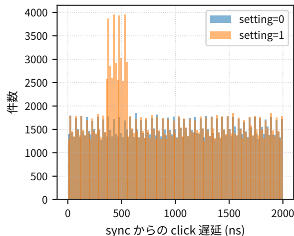
Alice : click 遅延 と setting
