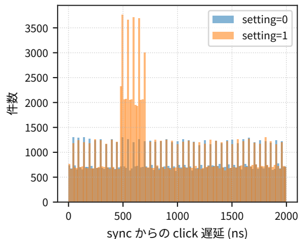
Bob : click 遅延 と setting
