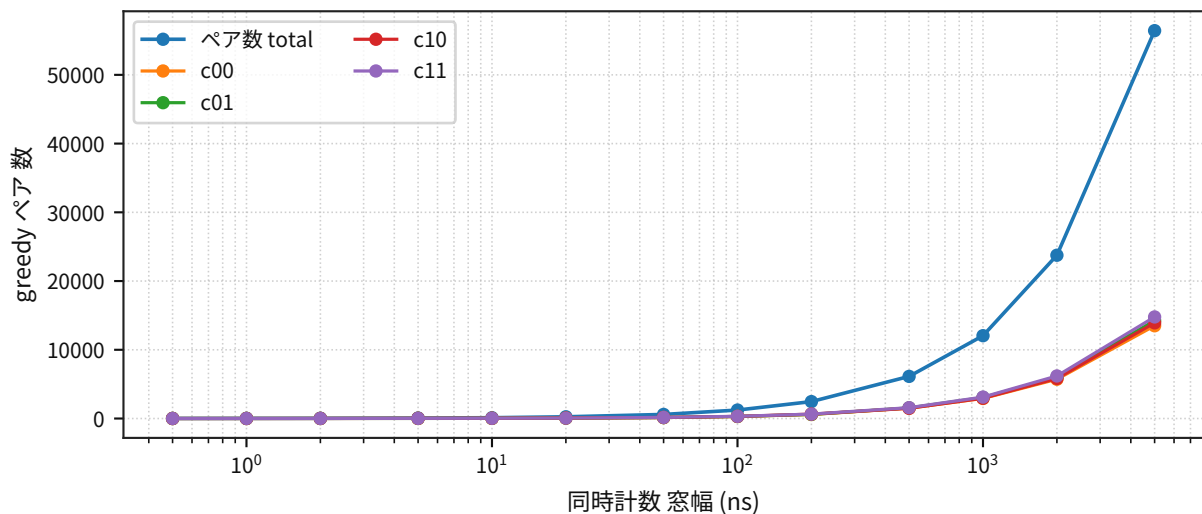
窓幅依存 (GPS PPS 整列)
