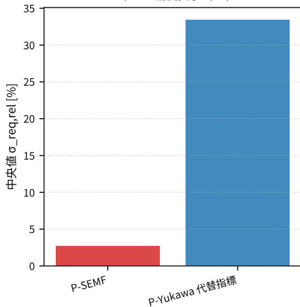
チャンネル精度要求 ( 3\sigma )
