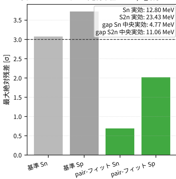
独立クロスチェック (電荷半径キंक, A_{\text{最小}}=100 )
