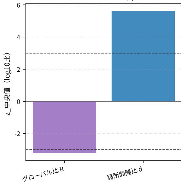
中央値残差の整合性 ( |z| \leq 3 )
