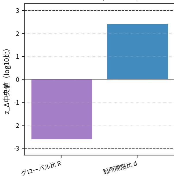
Aトレンド整合性 ( |z_{\Delta} \text{中央値}| \leq 3 )
