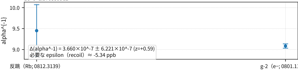
\alpha 精度クロスチェック
