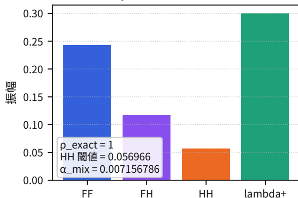
q_{\text{theory}} におけるランク1閉包
