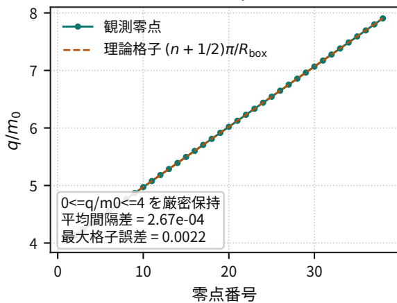
符号交代: 高 q 零点格子
