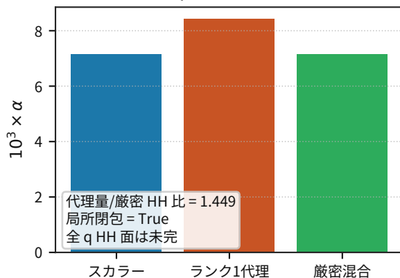
固定 q における \alpha 支持
