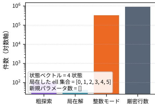
数値解法とスペクトルの尺度
