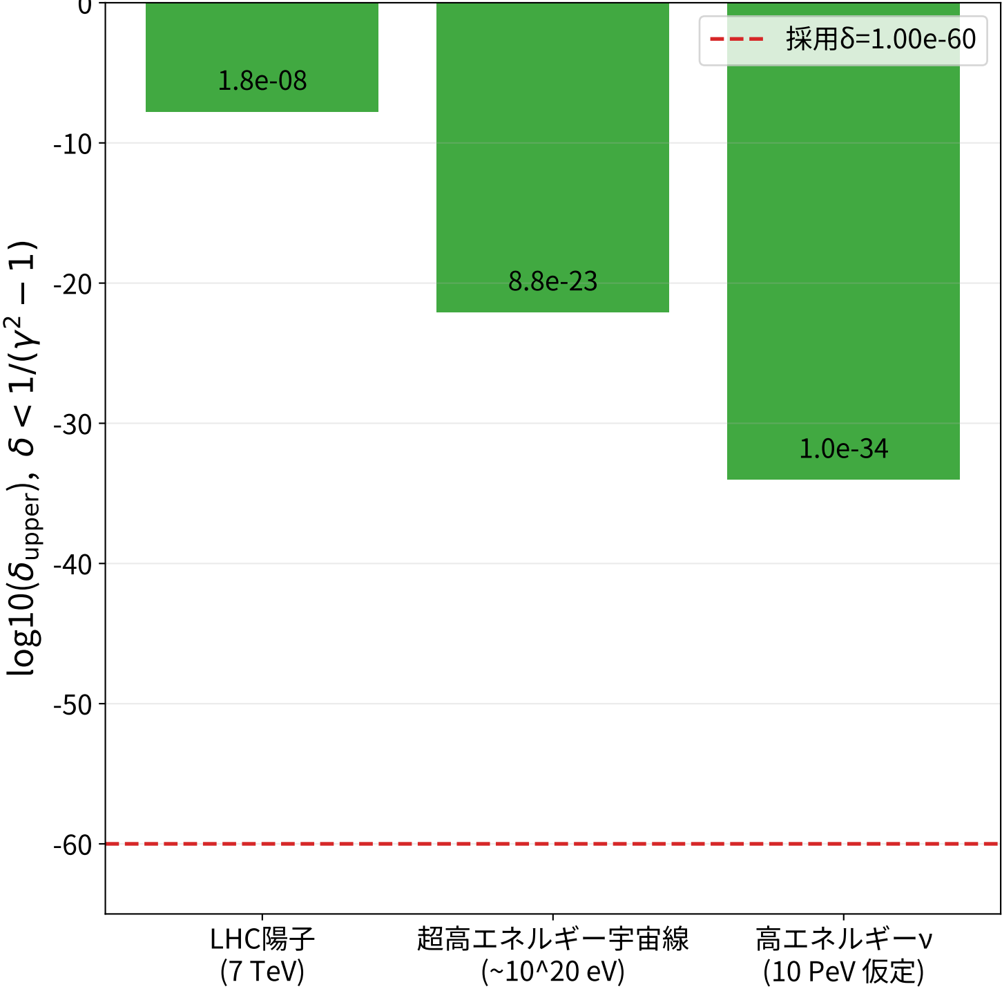
既存観測からの \delta 上限（概算）
