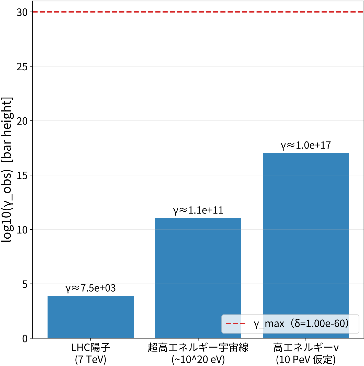
既存観測で到達しているローレンツ因子 \gamma
