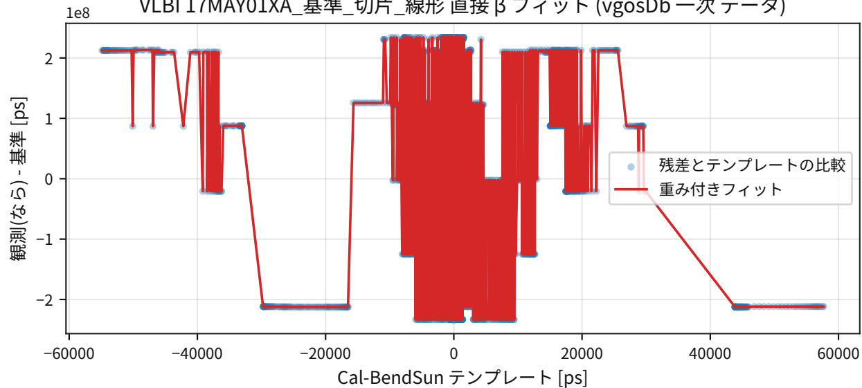
VLBI 17MAY01XA_基準_切片_線形 直接 \beta フィット (vgosDb 一次 データ)
