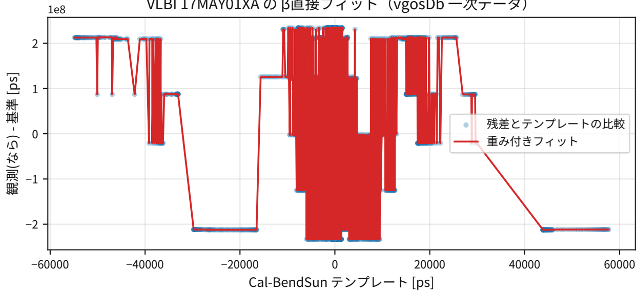
VLBI 17MAY01XA の \beta 直接フィット (vgosDb 一次データ)
